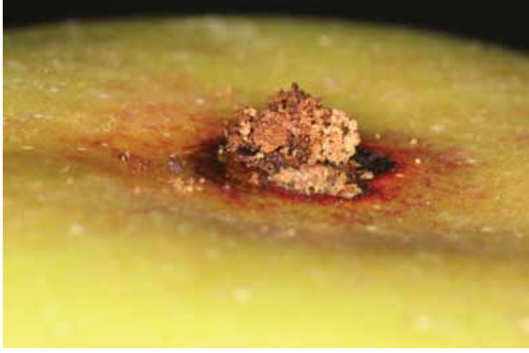
Owocówka jabłkowiec, objawy żerowania Cydia pomonella
