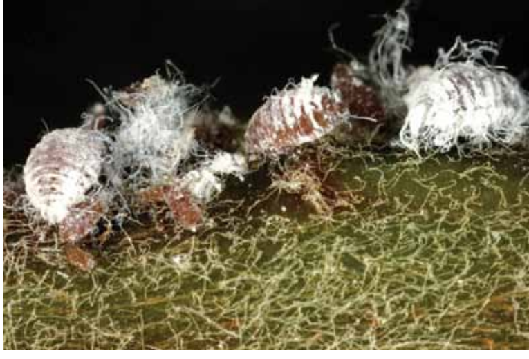
Bawełnica korówka, osobniki dorosłe Eriosoma lanigerum
